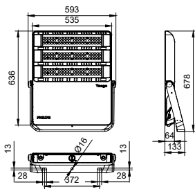
BVP384 LED565/WW 490W 220-240V AMB GM
